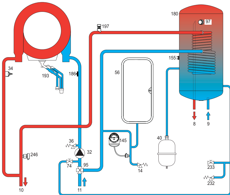
fig. 48- Circuito hidráulico
