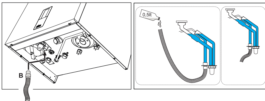
εικ. 37- Σύνδεση εξαγωγής συμπυκνώματος
