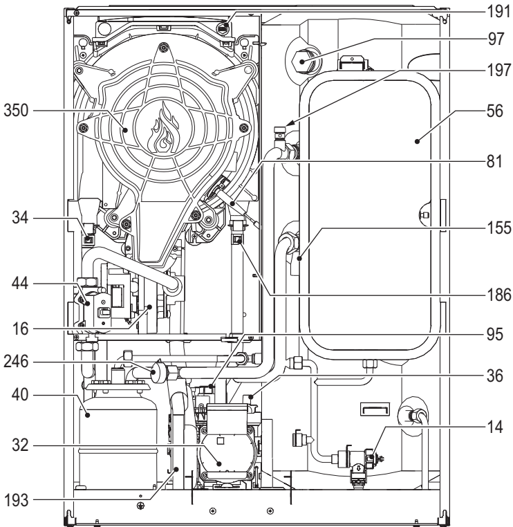
fig. 47- Vedere generală
