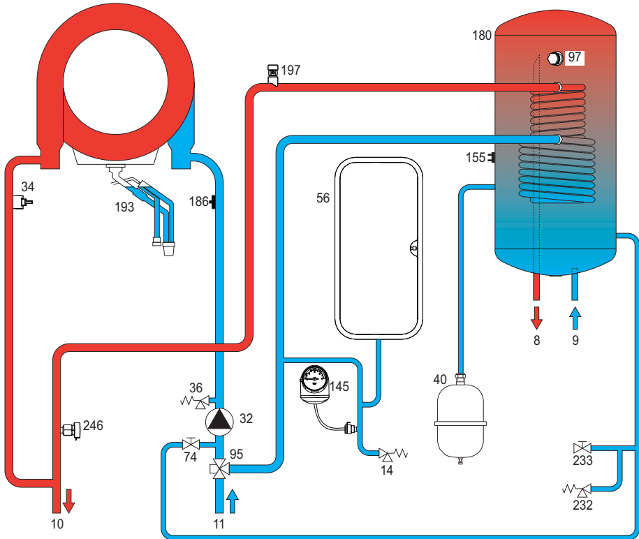
fig. 48 - Circuito idraulico
