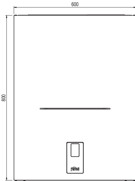
wygląd 43- Widok z przodu
