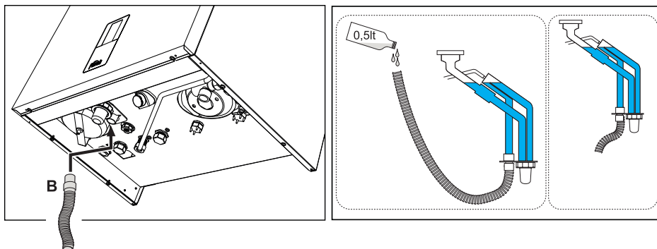
wygląd 37- Podłączenie spustu kondensatu
