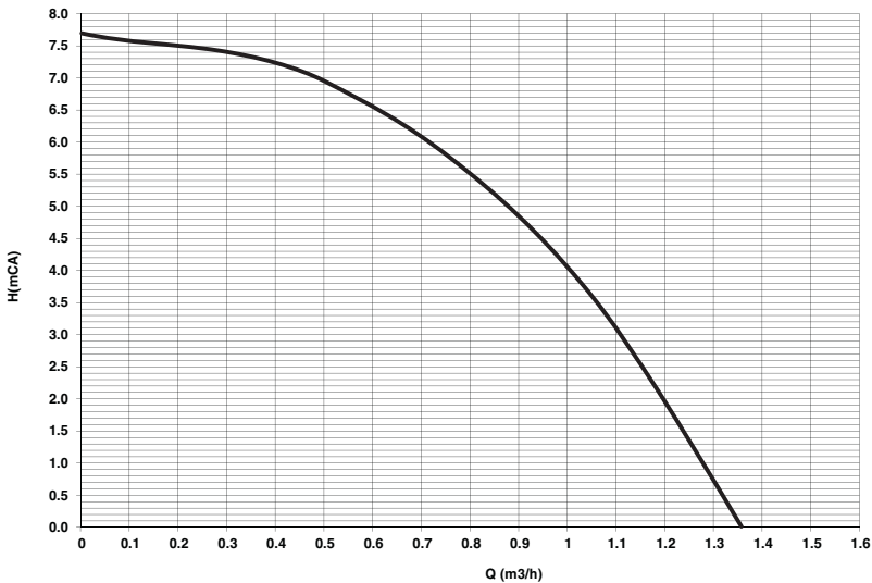
εικ. 50- Διαθέσιμο υπολειπόμενο μονομετρικό ύψος στην εγκατάσταση
