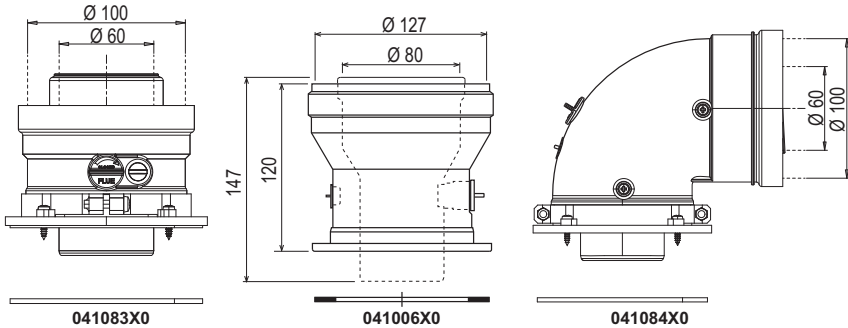
fig. 31 - Accessori di partenza per condotti coassiali
