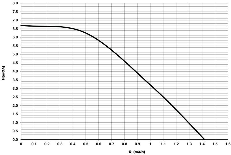
wygląd 49- Wysokość podnoszenia dostępna w instalacji
