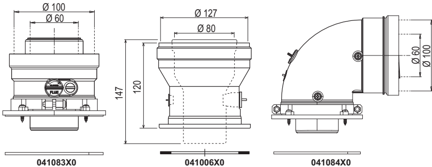
wygląd 31- Akcesoria wyjściowe do przewodów współosiowych
