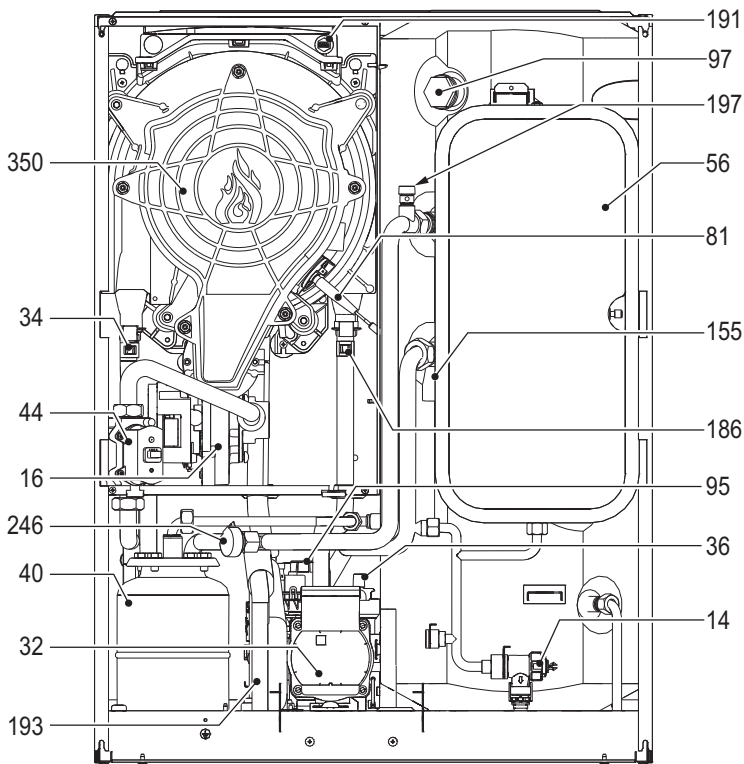
εικ. 47- Γενική όψη
