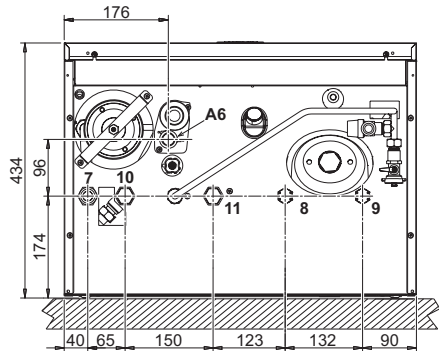
fig. 46 - Vista dal basso
