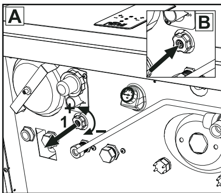
εικ. 26- Διακόπτης πλήρωσης
