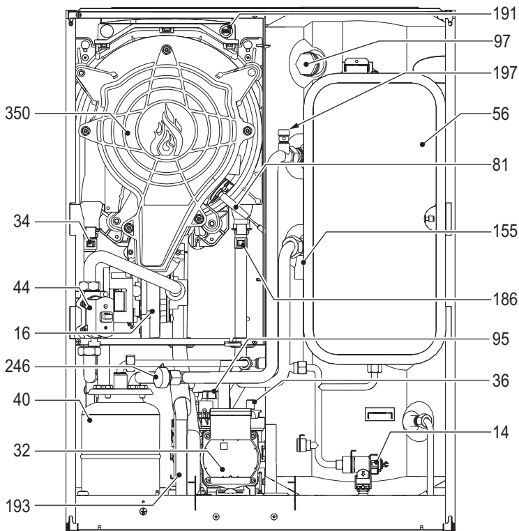
wygląd 47- Widok ogólny
