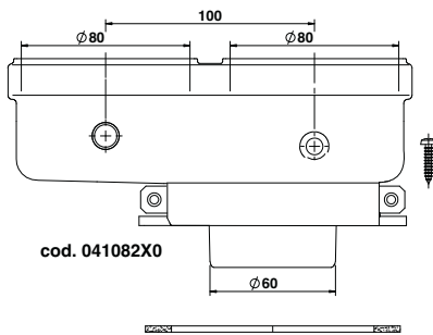
fig. 33 - Accessorio di partenza per condotti separati
