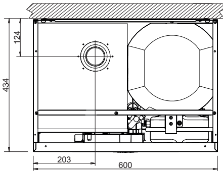
εικ. 45- Κάτωψη
