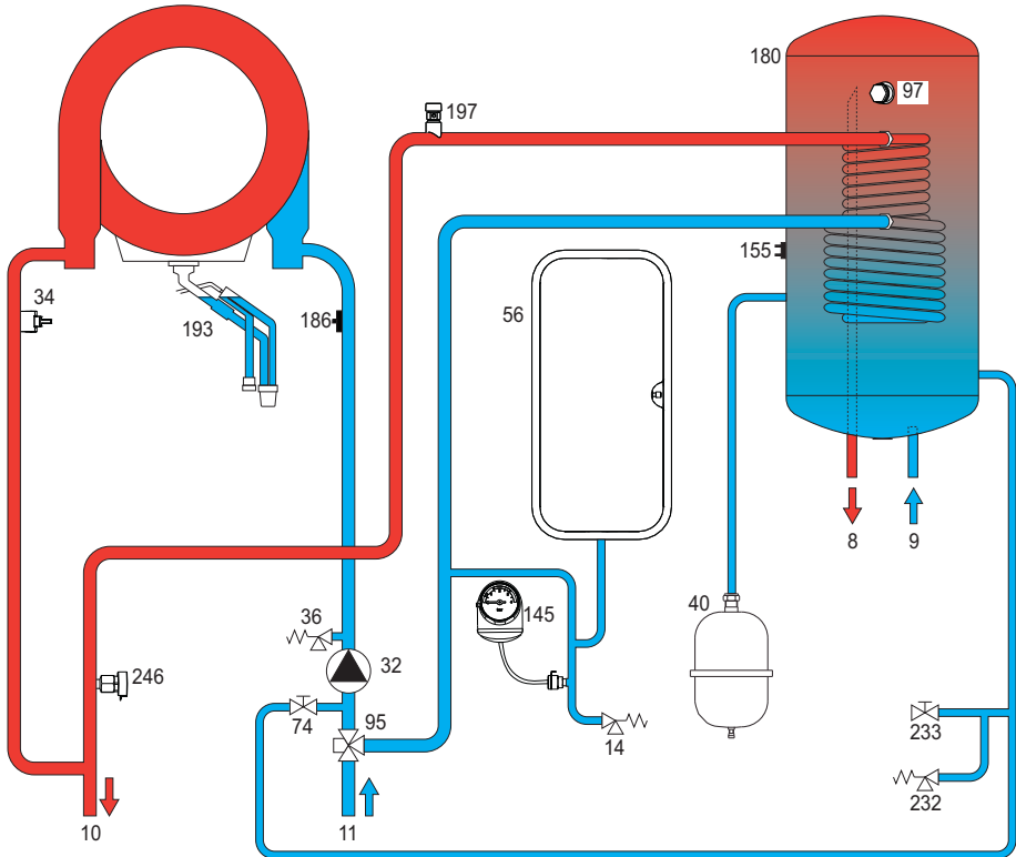
εικ. 48- Υδραυλικό κύκλωμα
