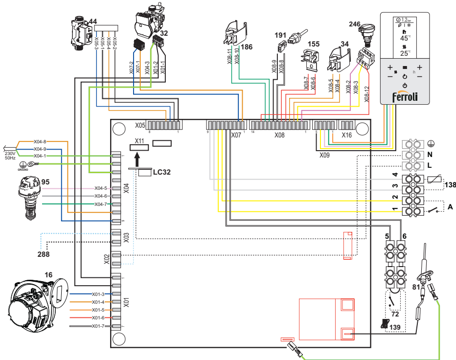
fig. 51 - Schema elettrico
