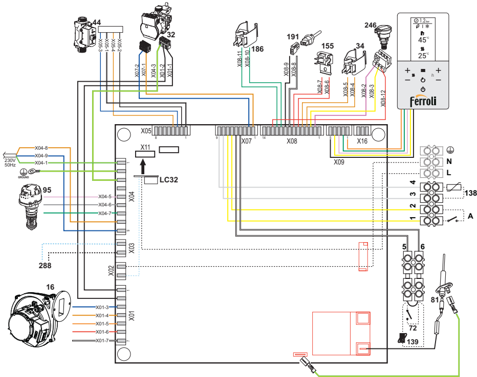
wygląd 51- Schemat instalacji elektrycznej
