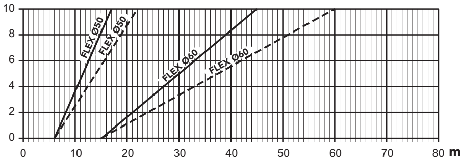
fig. 35 - Grafico per scelta parametro camino
