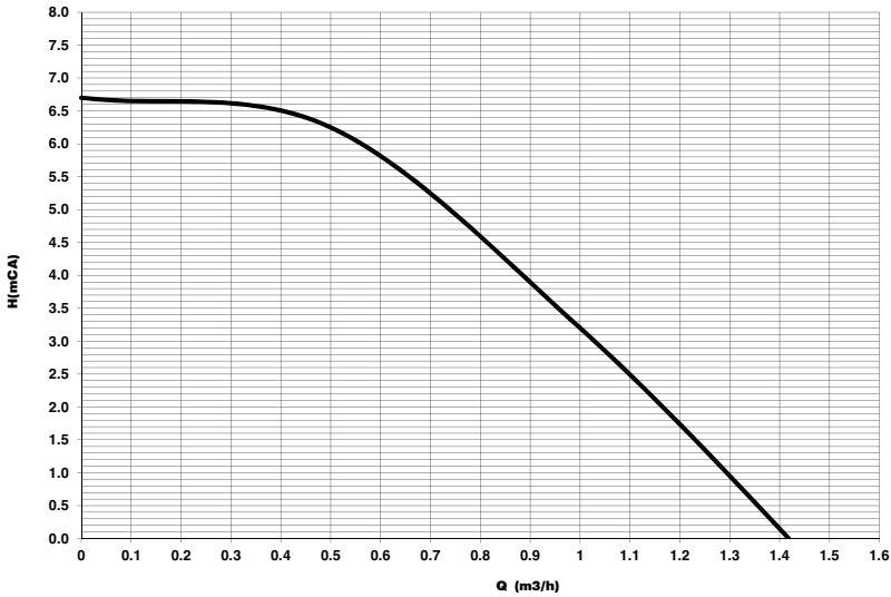
fig. 49 - Prevalenza residua disponibile all'impianto
