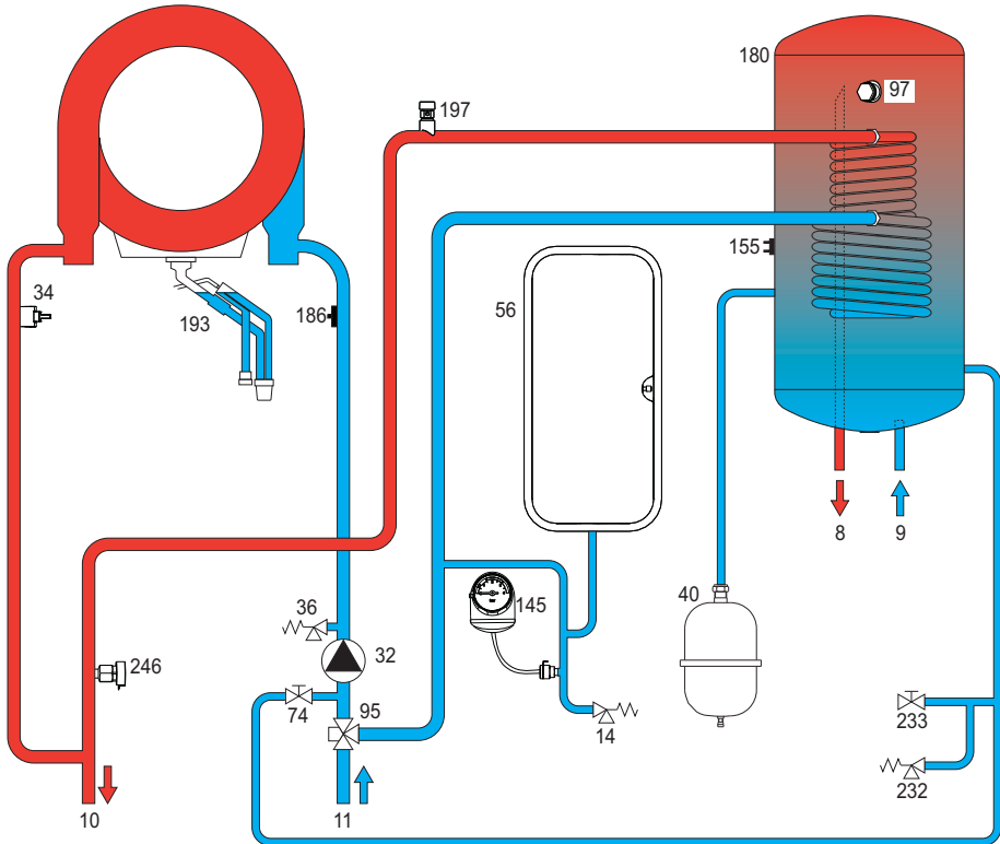
wygląd 48- Obieg wody
