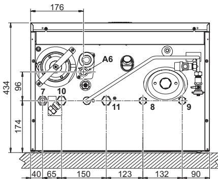
fig. 46- Vista inferior
