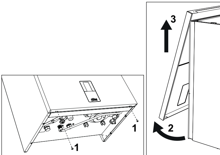
εικ. 41- Άνοιγμα μπροστινού πίνακα
