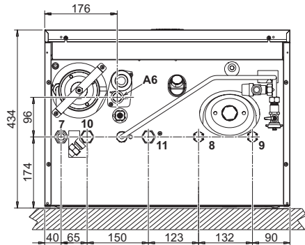
wygląd 46- Widok od dołu
