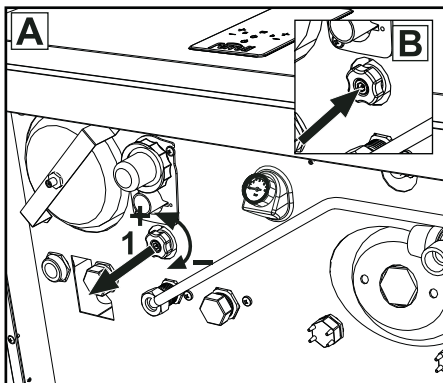
fig. 26- Filling knob
