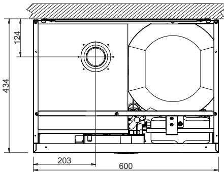
wygląd 45- Widok z góry
