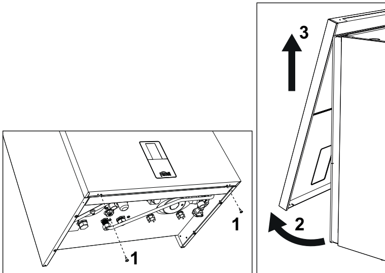
fig. 41 - Apertura pannello frontale
