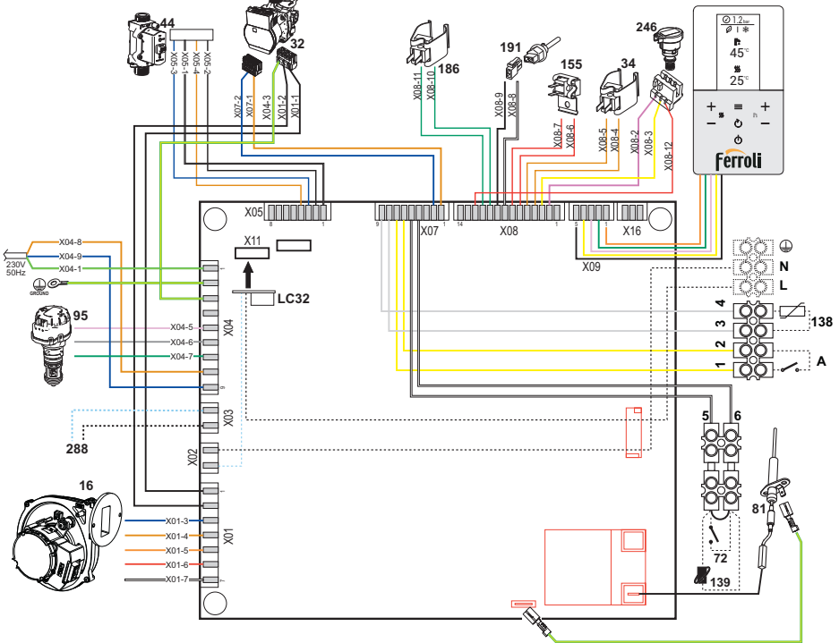
fig. 51- Esquema eléctrico
