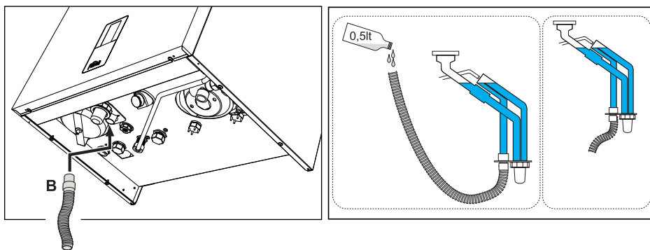
fig. 37 - Collegamento scarico condensa
