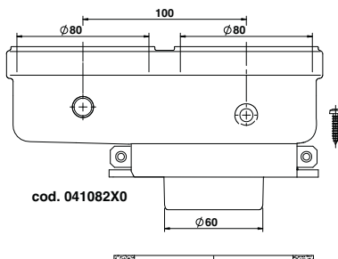
wygląd 33- Człon początkowy do montażu oddzielnych przewodów
