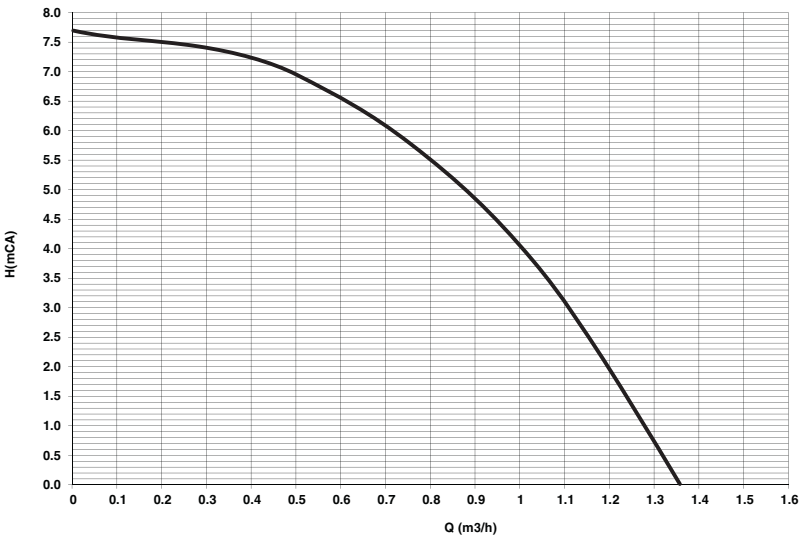
wygląd 50- Wysokość podnoszenia dostępna w instalacji
